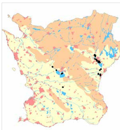
Figur 2. Gullstånds i Skåne (och Norden) 1989–2005 enl. Floran i Skåne. Arterna och deras utbredning (Tyler m.fl. 2007).
