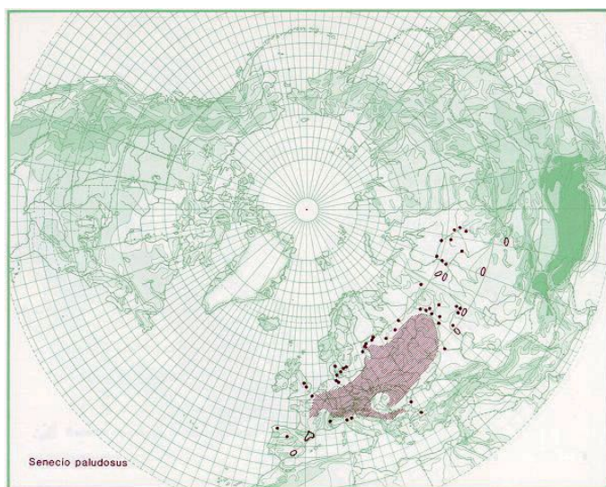
Figur 1. Utbredningen för gullstånds i Norden och världen enl. Hultén 1971 och Hultén & Fries 1986.
