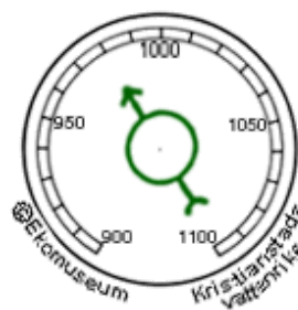
Lägsta lufttryck 982,2 hPa (den 4/2 2003 c:a kl 1:00)
