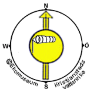
Maxvind Sydlig frisk vind 12,1 m/s (den 2/2 2003 c:a kl 17:00) ( beskrivning )
